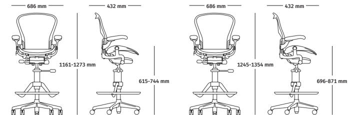
Hocker mit niedrigem Zylinder
