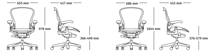
Bürostuhl Größe A
