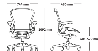
Bürostuhl Größe C
